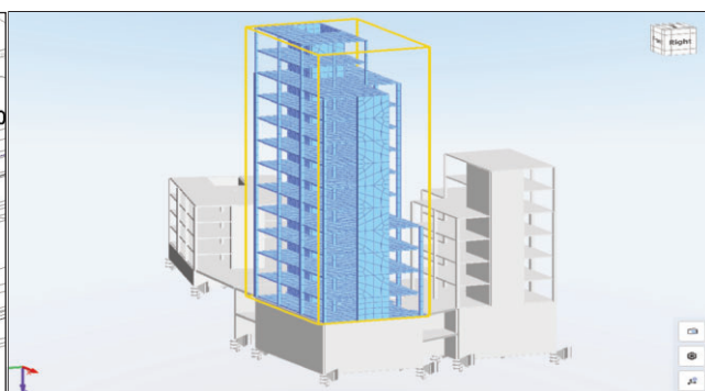
SOFiSTiK Erdbebenberechnung
