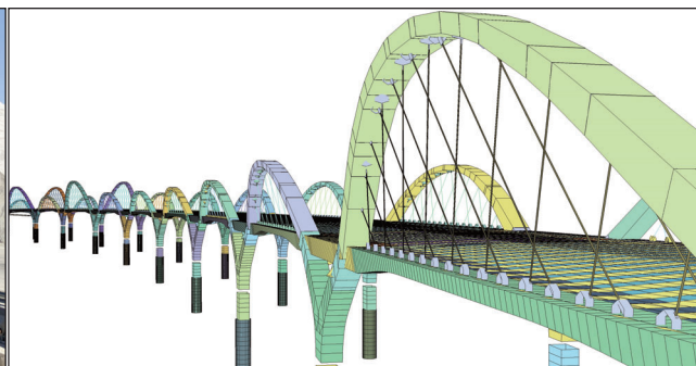
SOFiSTiK BIM-Rechenmodell
